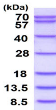
15% SDS-PAGE (5ul)
